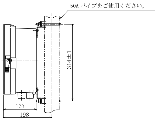
EFM204AWM 形 電磁流量計式水道メーター変換器寸法図
